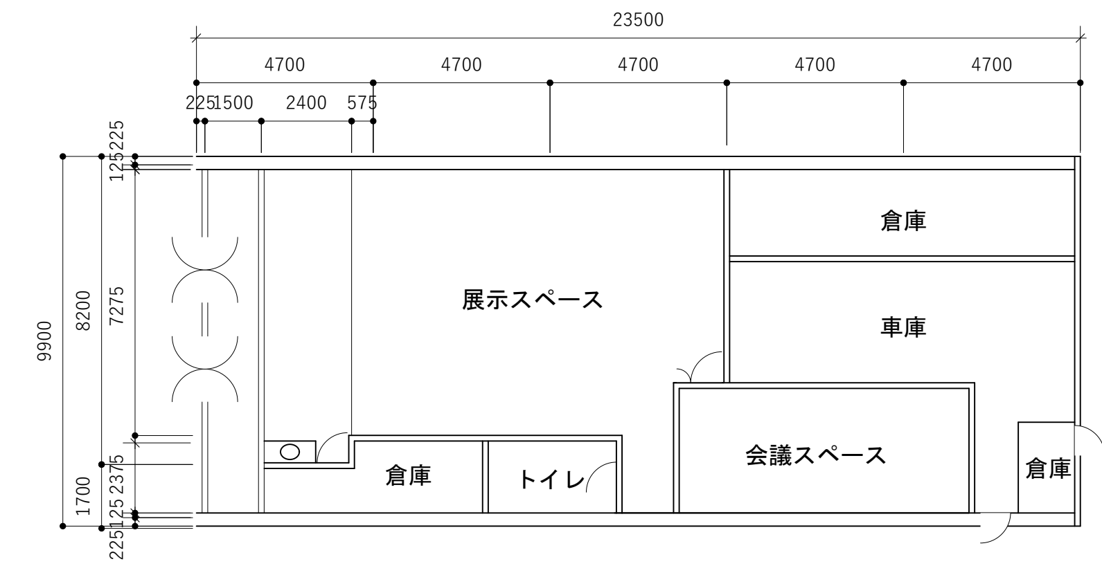
-現況平面図-
