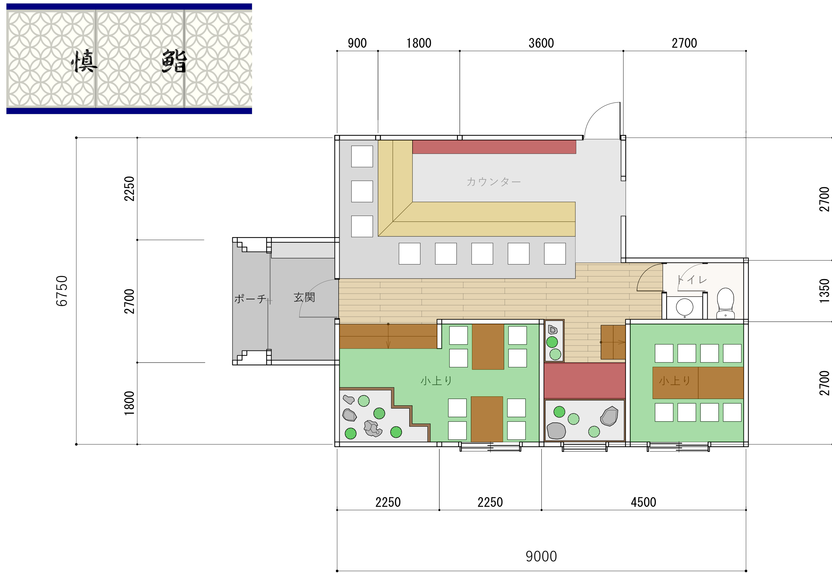
1階店舗平面図 1/100
