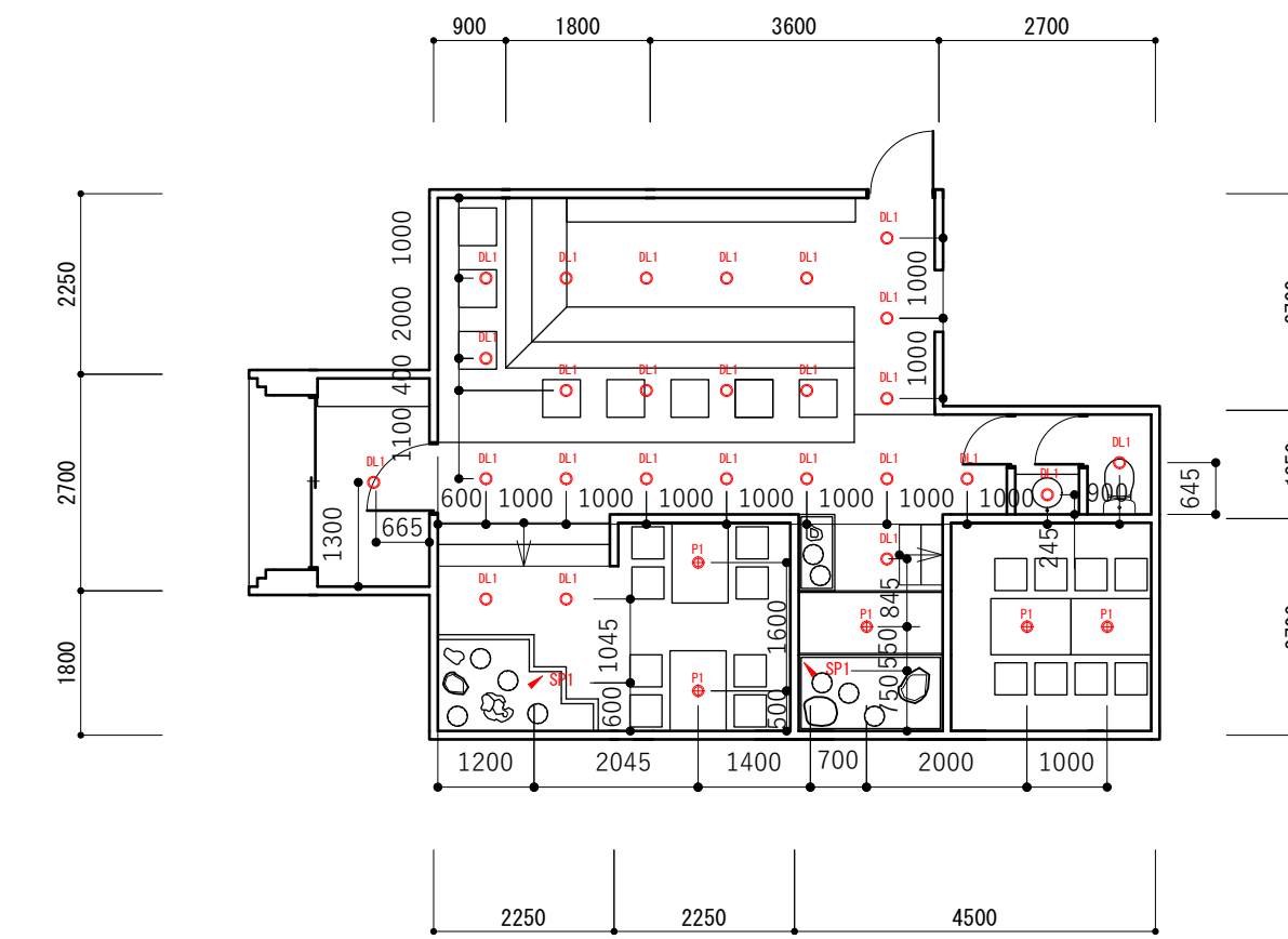
1階店舗天井伏図 1/100
