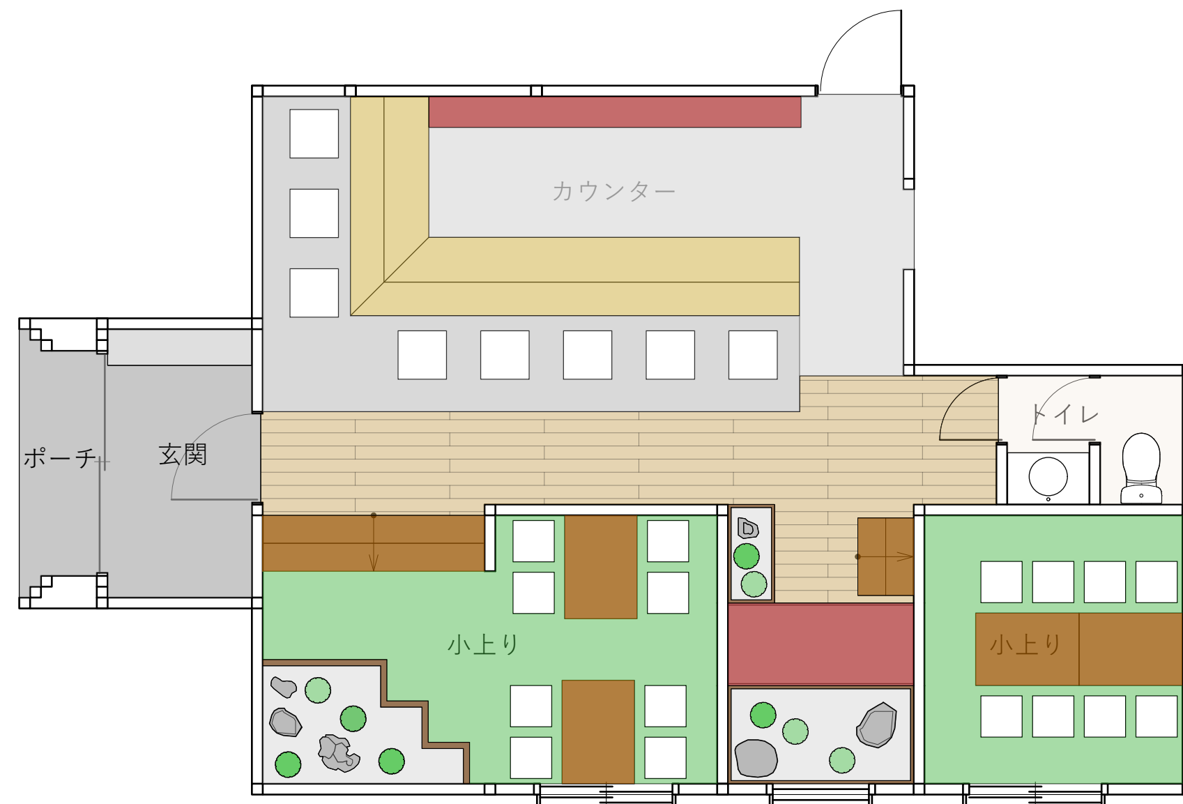
1階店舗平面図 1/100
