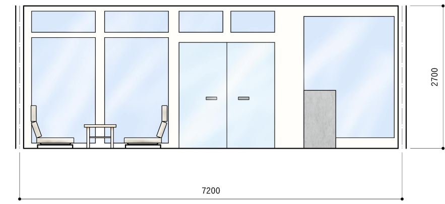
展開図A面 S=1/50
