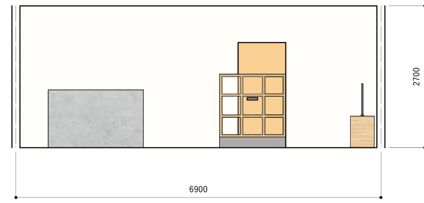
展開図B面 S=1/50
