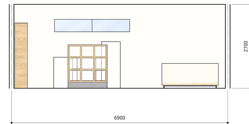
展開図D面 S=1/50
