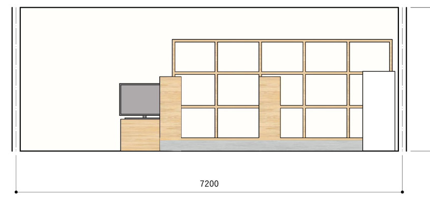
展開図C面 S=1/50
